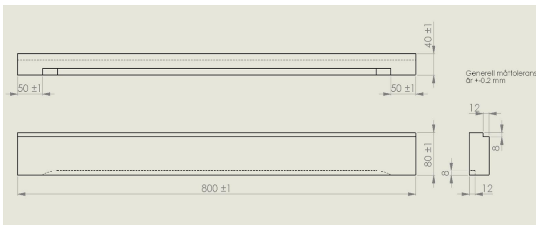
Skiss till praktikprov bordsfräs, fräsa mot anhåll
