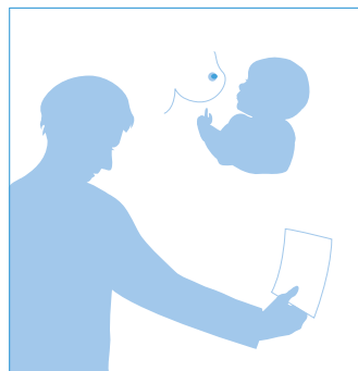
Figur 7. Närpunkten flyttas allt längre bort med ökande ålder.
