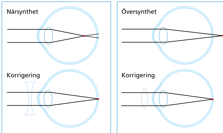
Figur 4. Vid närsynthet (till vänster) hamnar avbildningen av avlägsna föremål framför näthinnan. Fokalpunkten flyttas bakåt till näthinnan med hjälp av glasögon eller kontaktlinser med negativ brytkraft. Föremål på nära avstånd avbildas däremot korrekt på näthinnan utan glasögon. Vid översynthet (till höger) hamnar avbildningen av avlägsna föremål bakom näthinnan. Föremål på långa avstånd kan avbildas korrekt men detta kräver att linsmuskeln aktiveras för att anpassa linsens brytkraft till avståndet (ackommodation). Fokalpunkten flyttas framåt till näthinnan med hjälp av glasögon eller kontaktlinser med positiv brytkraft.
