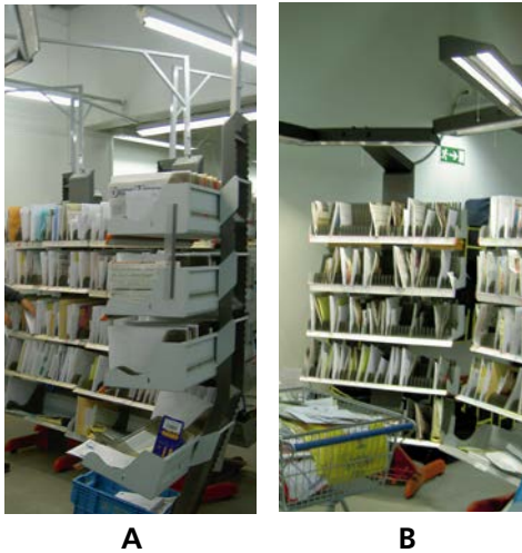
Figur 66. Postsorteringshyllor före (A) och efter (B) montering av asymmetrisk belysning.
