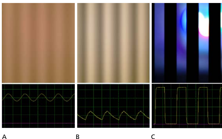
Figur 21. Exempel på hur en ljuskällas ljusmodulation kan analyseras grovt med ett mobilfoto:
