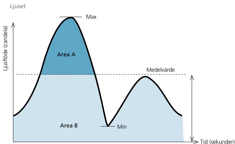
Figur 20. Ljusflöde under en flimmericykel. Flimmerprocent beräknas som (\text{Max} - \text{Min}) / (\text{Max} + \text{Min}) \times 100 . Flimmerindex beräknas som \text{Area A} / (\text{Area A} + \text{Area B}) .
